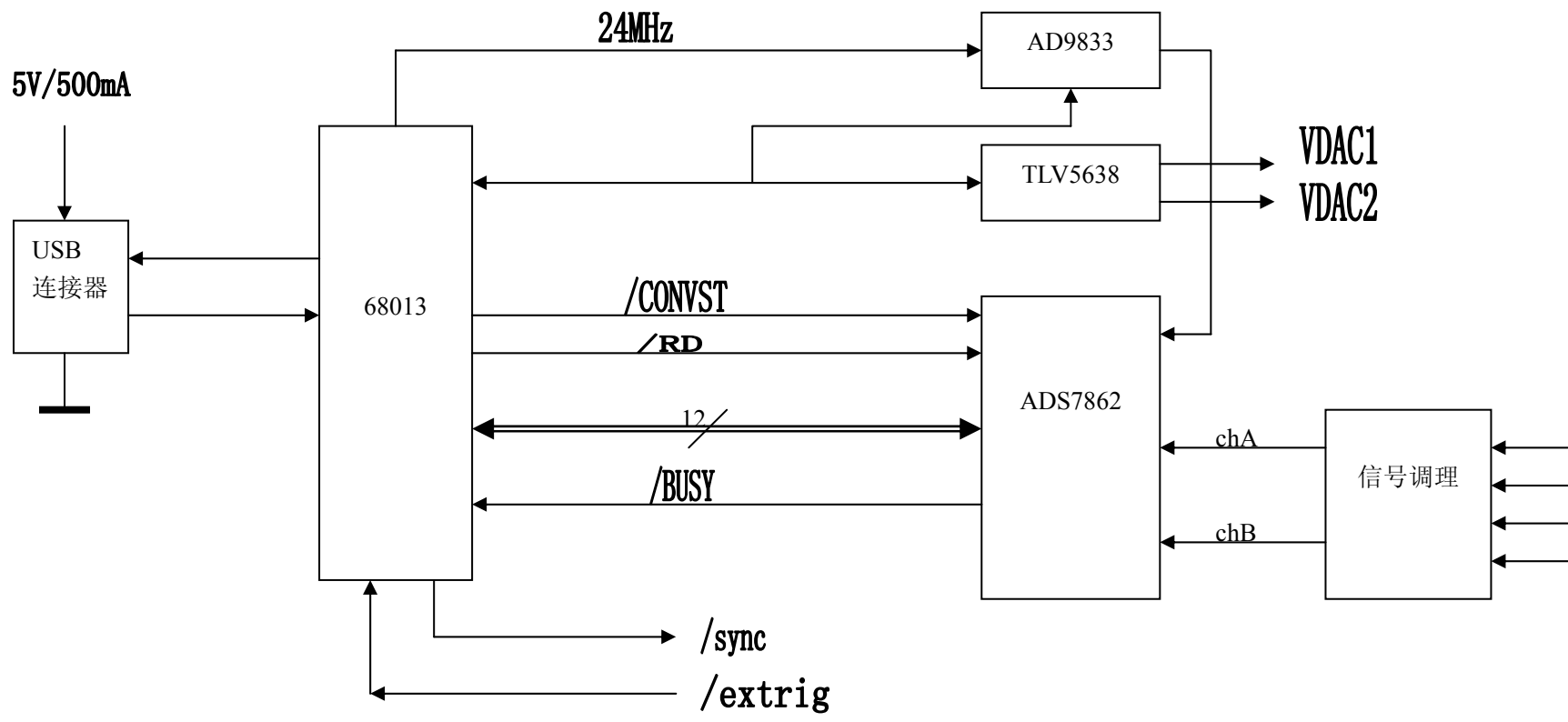
USB数据采集器原理框图
